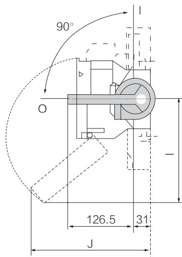
SXG1R-63~400-RCJ柜外侧面操作
