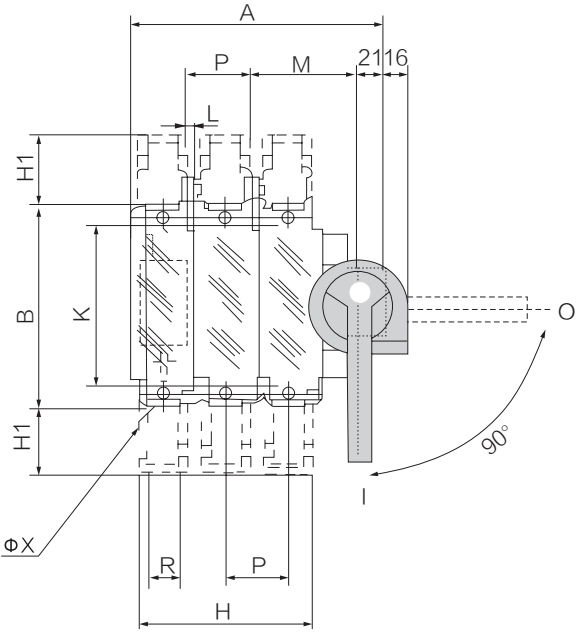
SXG1R-63~400-RJ柜外正面操作
