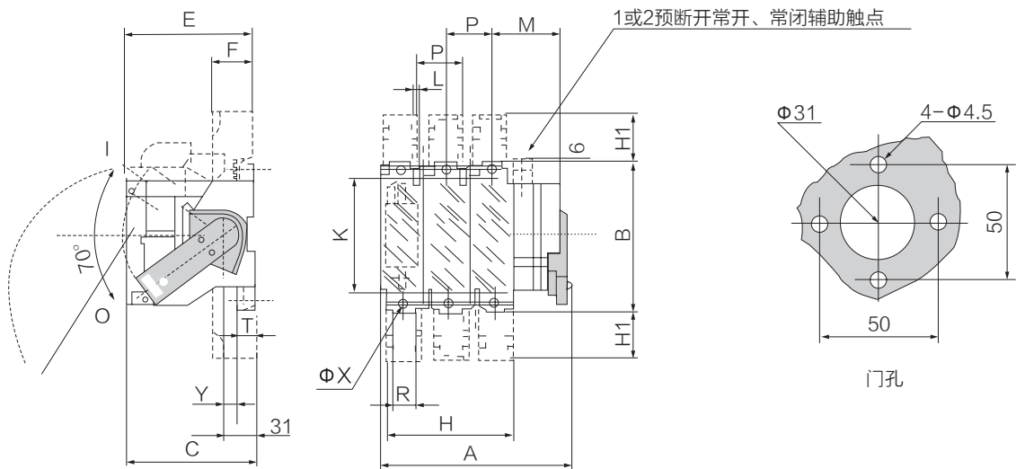
SXG1R-63~400-RC侧面操作
