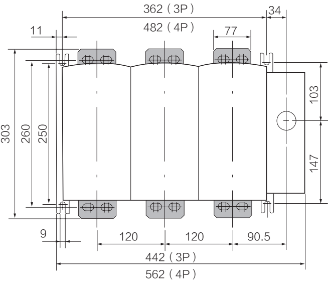
安装尺寸
